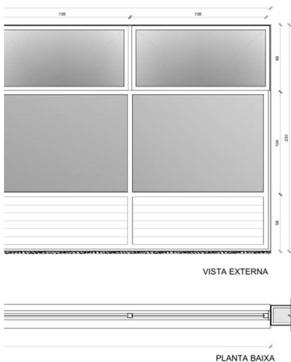
JA-08 JANELA TIPO FIXA COM BANDEIRA MAXIMAR QUANT.: 01 DIMENSÕES: 700 x 290 cm DETALHE: - K6
